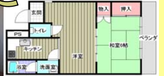
【工事前図面】
